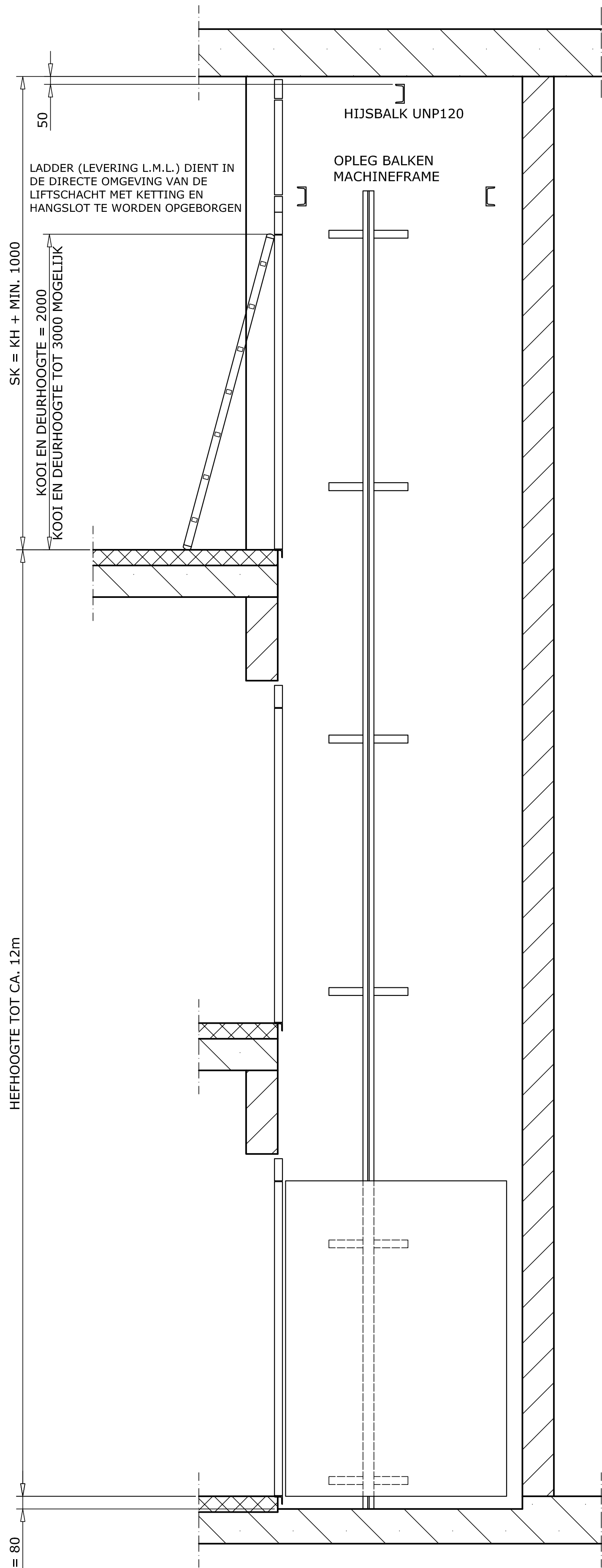
ZIJZICHT EN DOORSNEDE
