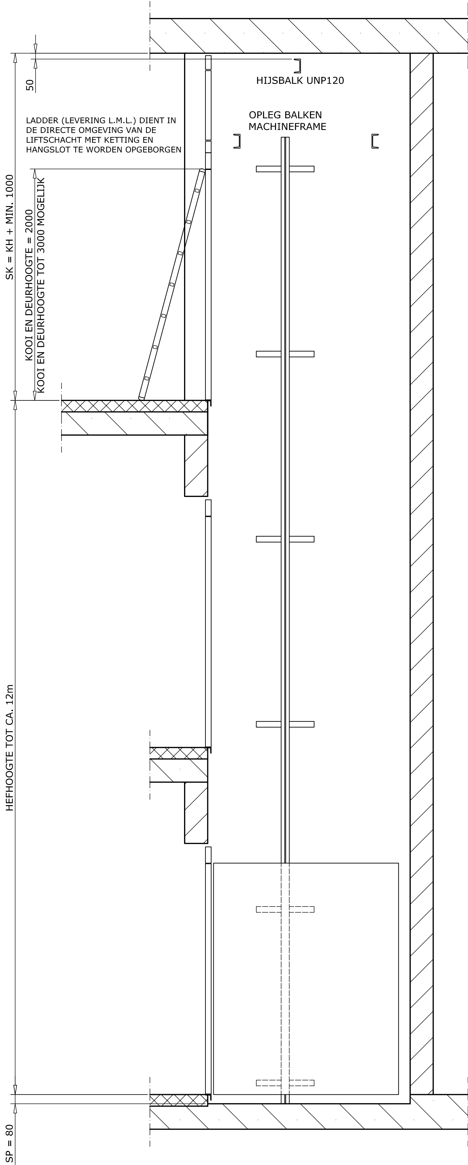
ZIJZICHT EN DOORSNEDE
