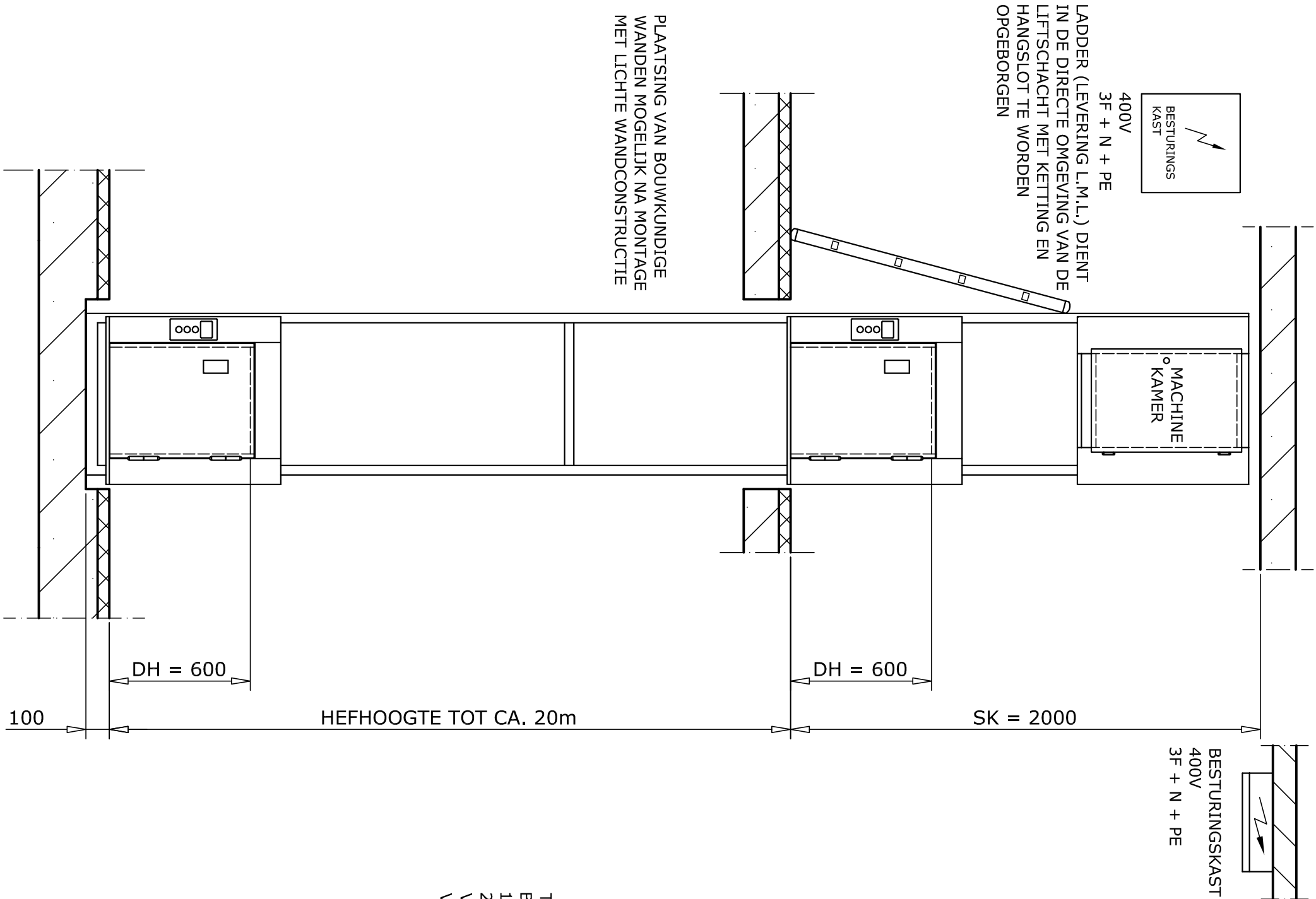
MACHINEKAMER GEÏNTEGREERD IN BOVENZIJDIGE SCHACHT
