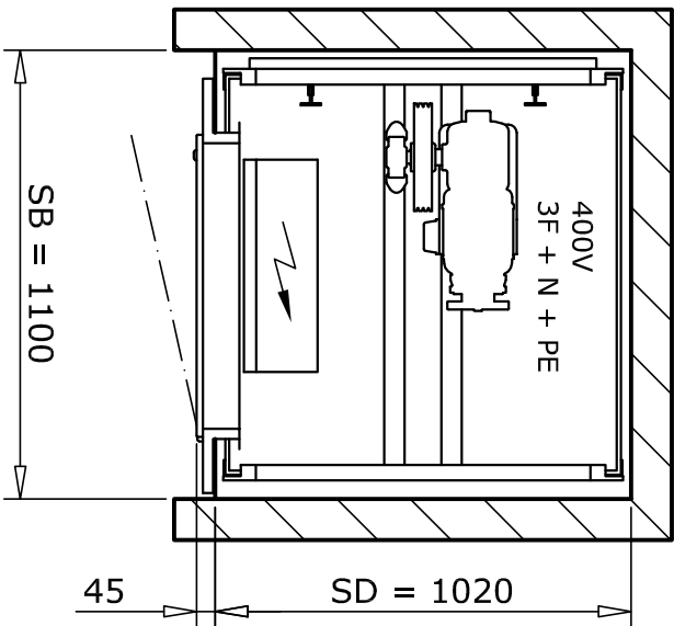
MACHINEKAMER GEÏNTEGREERD IN BOVENZIJD E SCHACHT
