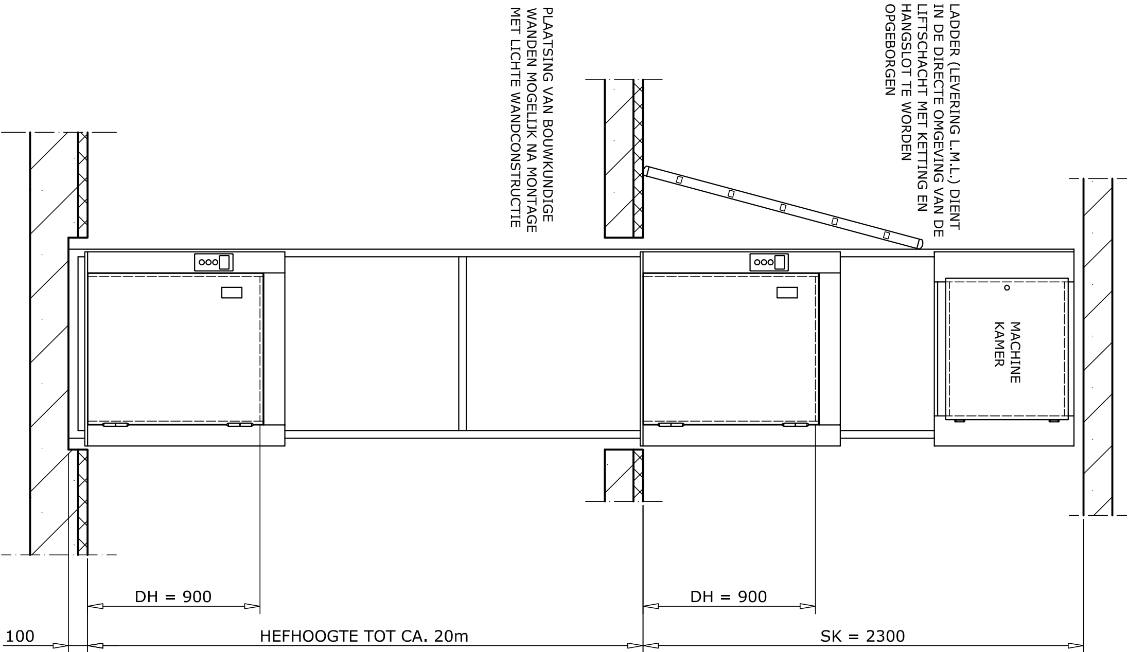
VOORAANZICHT EN DOORSNEDE
