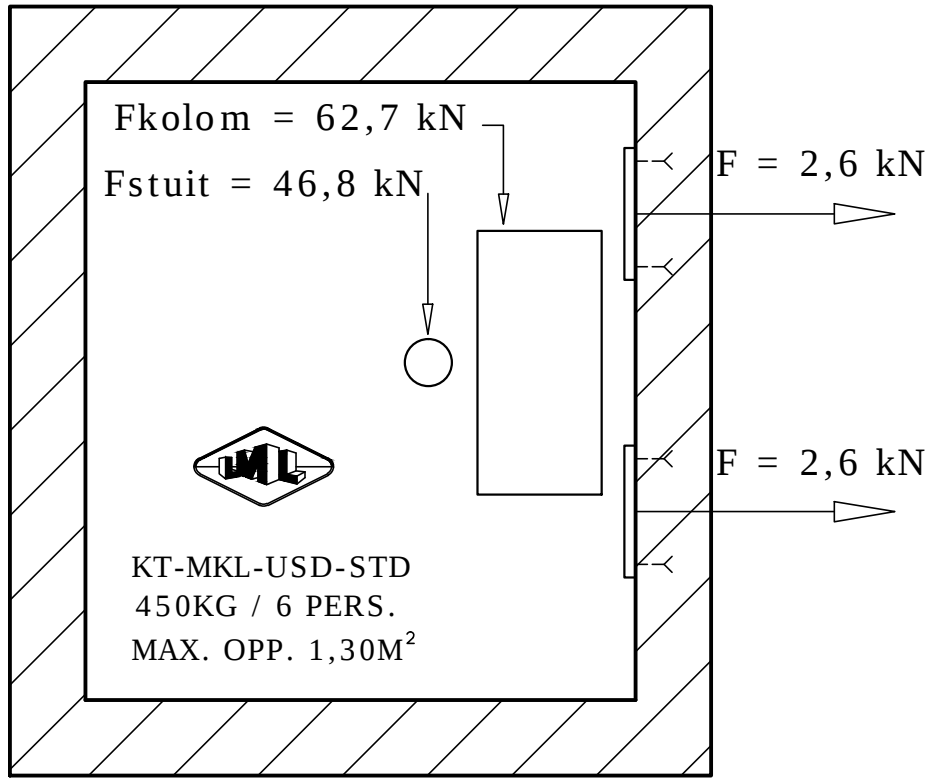
PUT- EN WANDBELASTING INDIEN USD UITVOERING 2 KOOSTUITEN Fstuit = 23,4kN PER STUIT
