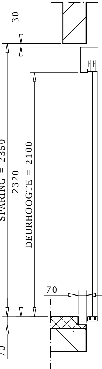
DOORSNEDE TOEGANG
