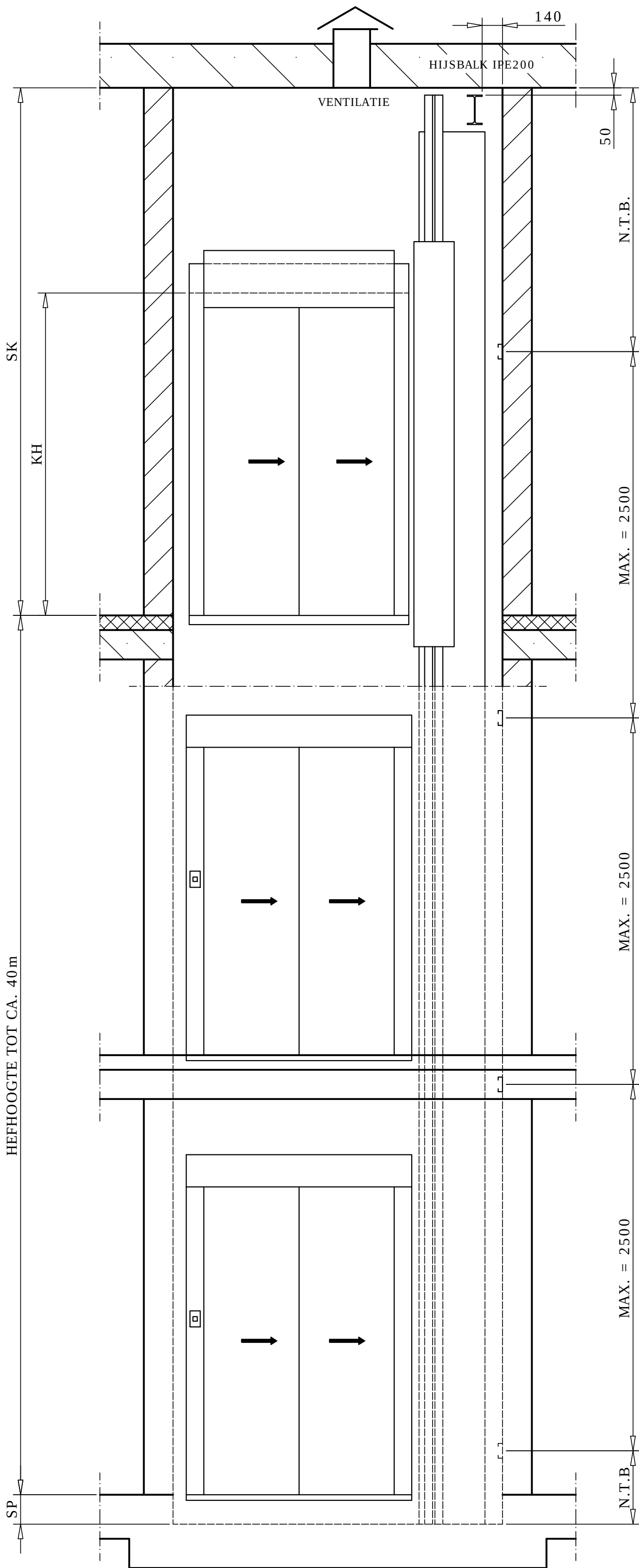
VOORAANZICHT EN DOORSNEDE
