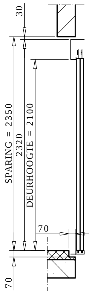
DOORSNEDE TOEGANG
